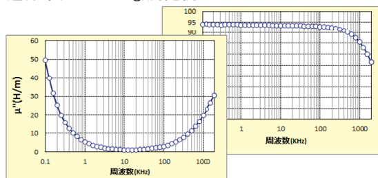
透磁率(Real/Imag)測定例
