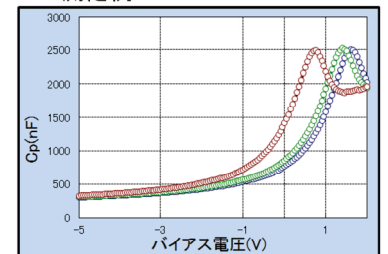
C-V測定例
