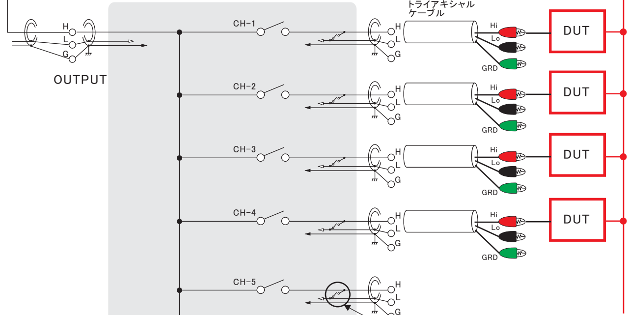
スキャナカード 6522/6521
