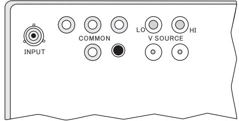
6517Aリアーパネル
