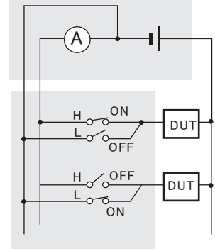
等価回路
