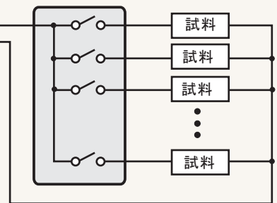
6517A内臓型スキャナカード 6521(30V/500mA),6522(200V/500mA)
